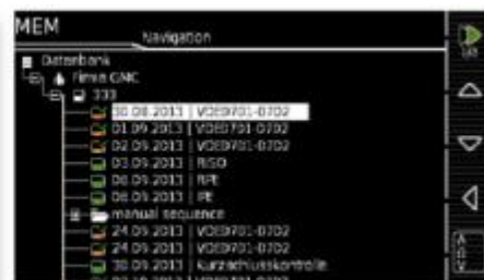
Database structuur
